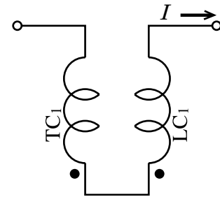
図 4 : 直列接続無誘導巻線限流器
