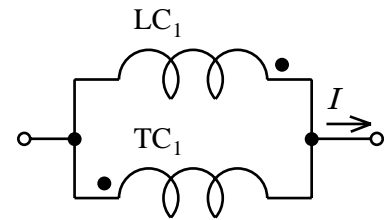
図 3 : 並列接続無誘導巻線限流器
