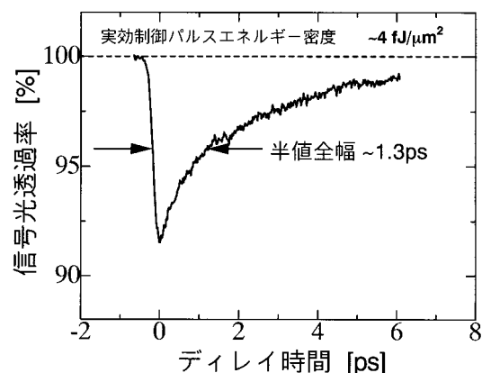
図2：光 光変調実験結果の一例
