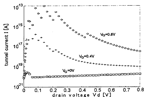
図2：I-V特性
