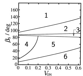
図3：動作モード分布図
