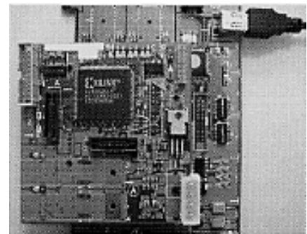
図2 リンク層LSIのFPGAによる実装
