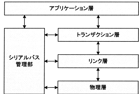
図1 IEEE1394デバイスの階層構造
