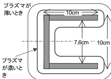
図1 プラズマ密度とシース形状
