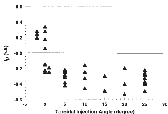
図2 ECHビーム入射角度とトロイダル電流 (0°はトーラス軸に対し垂直)
