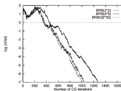
図2 ブロック化赤一黒順序付け法の収束性
