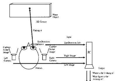
図2 装着型アクティブ・ビジョンセンサの構成
