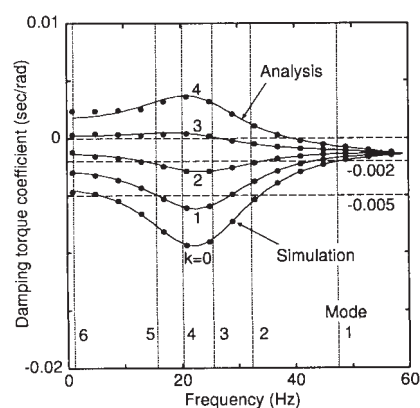
図3 点弧角制御の効果
