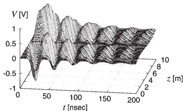
図8 導体1上の電圧分布
