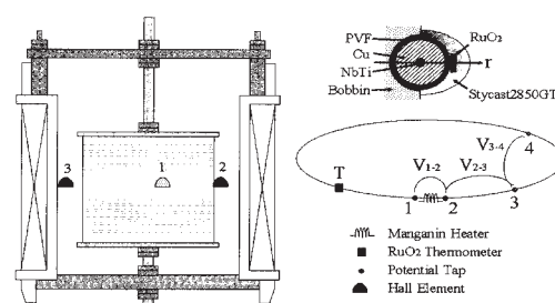
図2 試験体コイル、外部マグネットと測定点
