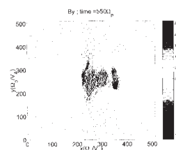
図2 t=550 （時間はプロトンジャイロ周期の逆数で規格化）の磁力線と同じ方向の磁場強度（磁力線成分を含む）
