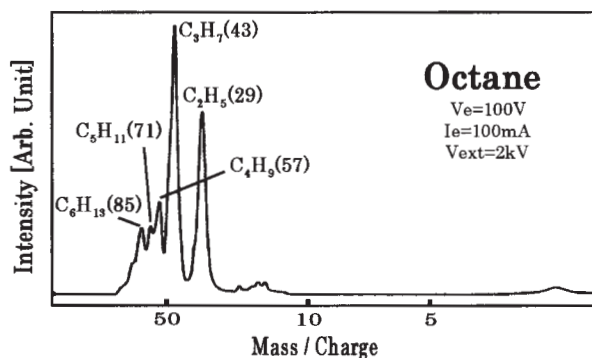
図2 オクタンイオンの質量分離特性
