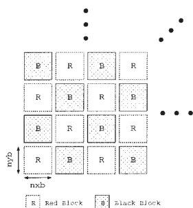
図1 ブロック化赤一黒順序付けにおけるブロック分割と色分け
