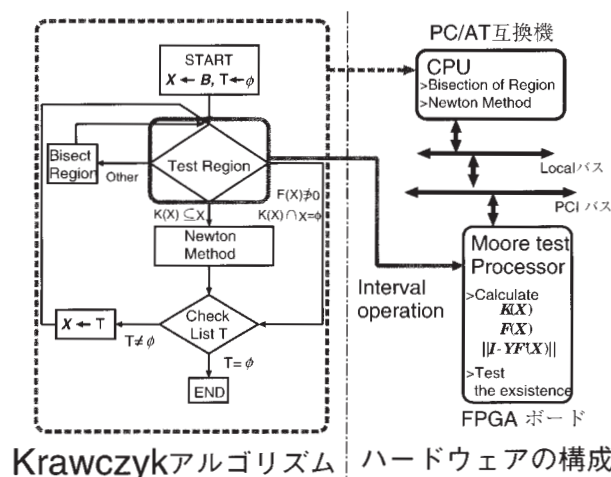
図5．アルゴリズムにおいてソフトで実行する部分とハードで実行する部分を分離。
