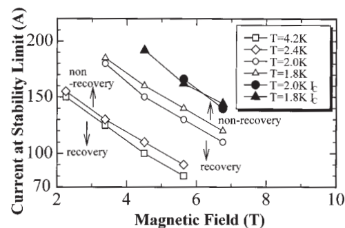
図3 安定限界電流の磁場及び液温依存性
