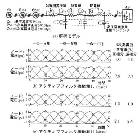
図2 提案制御方式による高調波拡大現象の抑制効果
