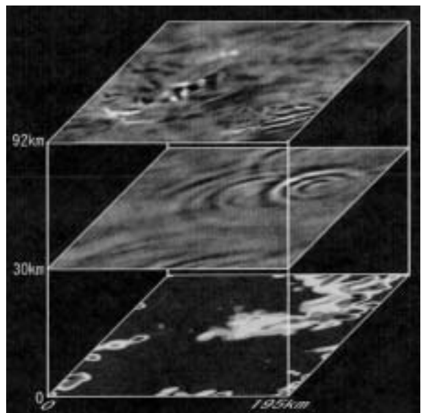
図 数値シミュレーション結果のスナップショット。地表における降水と、高度30, 90kmにおける鉛直風速。値のスケージングは両高度で異なり、30kmにおける鉛直風擾乱の振幅は1m/s以下であるのに対し、90kmでは数10m/sに達する。高度30kmでは重力波が波紋状に広がっている。90kmにおける右下隅の縞模様はより波長の大きい重力波の碎波による擾乱「リップル」である。
