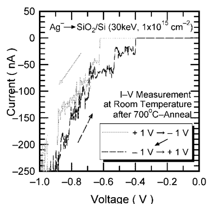
図2 銀超微粒子膜の電流・電圧特性
