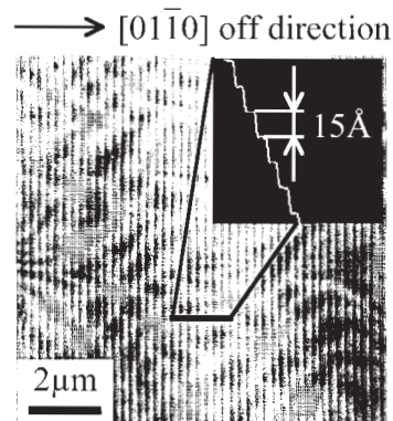
図 成長表面のステップ構造 (AFM像)
