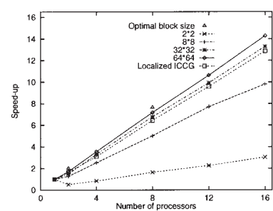
図3 ブロック化赤一黒順序付け法による速度向上
