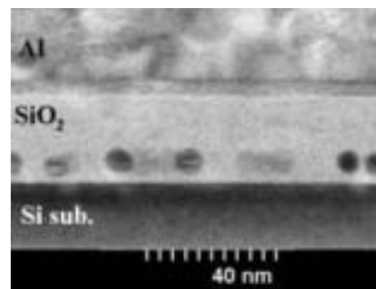
図3. SiO 2 薄膜底面に形成した単層銀ナノ粒子 (Ag - : 10 keV, 700℃アニール)
