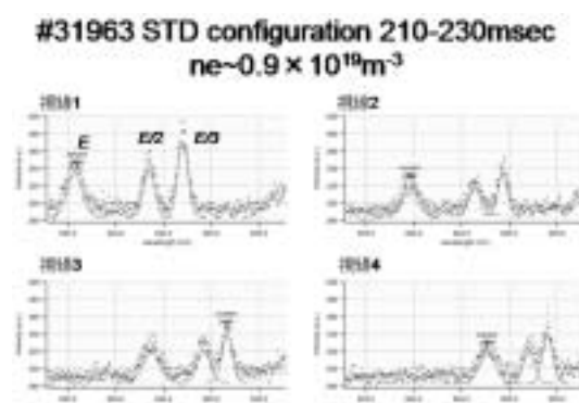
図2. 視線1～4で観測された H\alpha 光のベクトル
