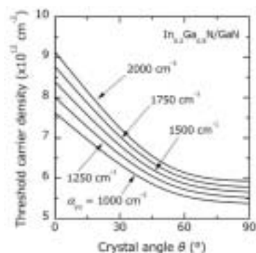
図2. InGaN LDにおけるしきい値キャリア密度の角度 \theta 依存性。
