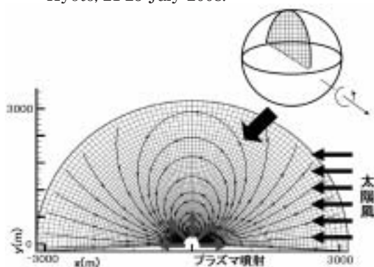
図1. 宇宙機からのプラズマ噴射モデル
