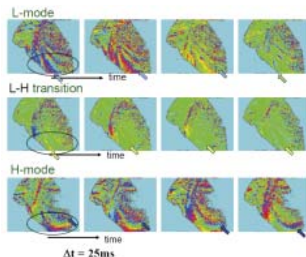
図5. 接線方向に撮影された画像データの二次元位相図の例(ECHプラズマ)。閉じ込め状態の異なる時間帯で、フィラメント構造の移動方向が異なっている。
