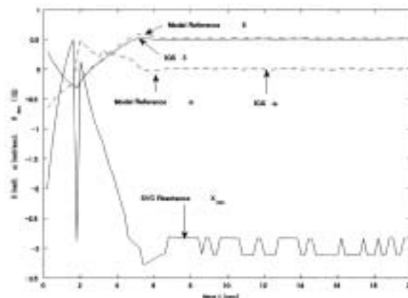
図2. SVC制御による発電機動揺抑制
