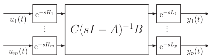
図1. 複数のむだ時間を含む多変数系( H_i : 入力むだ時間、 L_j : 出力むだ時間、 A, B, C : システム行列)
