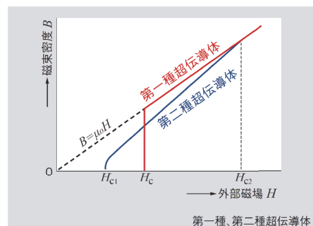
図2 第一種・第二種超伝導体の外部磁場と超伝導体内の磁束密度の関係 [1]
