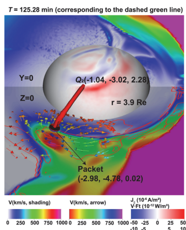
図 1：電磁流体シミュレーションで再現した惑星間空間衝撃波到来時の磁気圏。カナダ・ケベック州で大規模停電が発生した時刻に対応する。赤い線は、エネルギー（電流）の輸送を担うアルベン波の軌道を示す。
