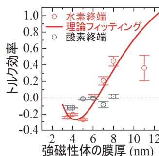
図2 トルク効率の強磁性体膜厚依存性。
