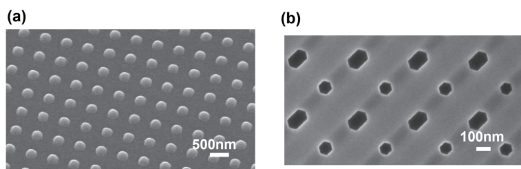
図1 (a)：薄膜シリコン系太陽電池の吸収効率増大のために作製したロッド構造、(b)：高ビーム品質・高出力青色レーザーに導入した GaN/ 空気孔ナノ構造
